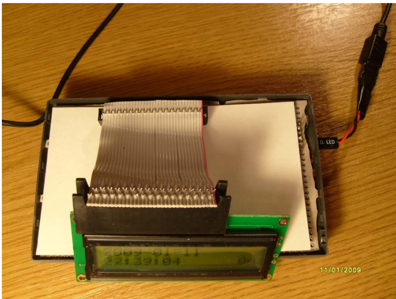
Slika 4: Informacijski zaslon tik preden sem prispajkal še LCD zaslon, Desno je viden pretvornik za USB kabel.
