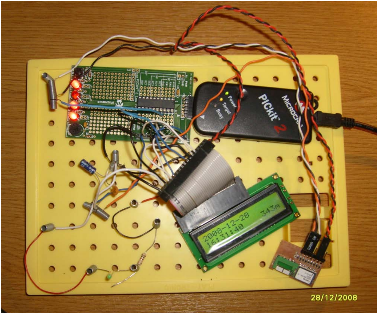
Slika 1: Prototip informacijskega zaslona. Zgoraj je viden programator PICkit 2, desno spodaj je GPS sprejemnik na bakreni ploščici.
