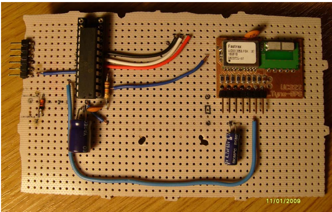
Slika 3: Zadnja stran informacijskega zaslona. Čisto na levi je 6 nožna letvica, kamor se priključi programator ali napajanje; levo je PIC mikrokontroler v podnožju, desno je GPS sprejemnik z anteno na dodatni bakreni ploščici.
